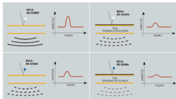
Respuesta al impacto de una losa de hormigón armado.
