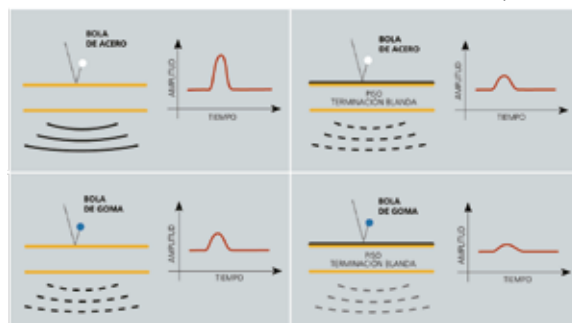
Respuesta al impacto de una losa de hormigón armado.
